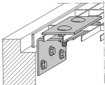
Gitterrostverschraubung
