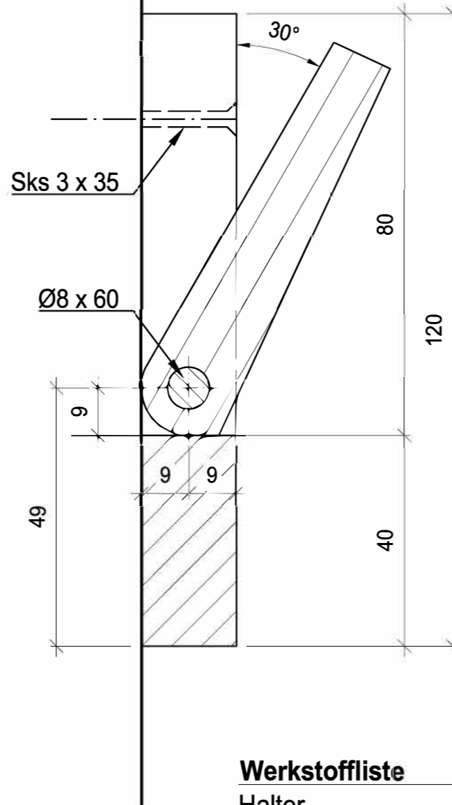
B-B
